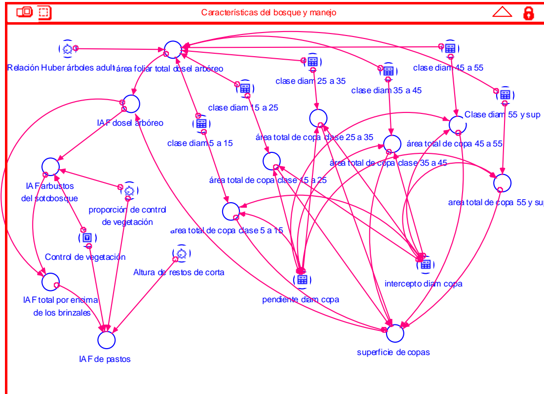
Figura 8: relaciones entre variables del módulo "Características del bosque y su silvicultura".
